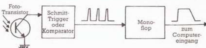
Bild 4. Einfaches Schaltungsschema des Lichtgriffels
